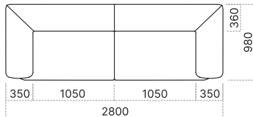
4-SEDÁK S 2 PODRUČAMI
